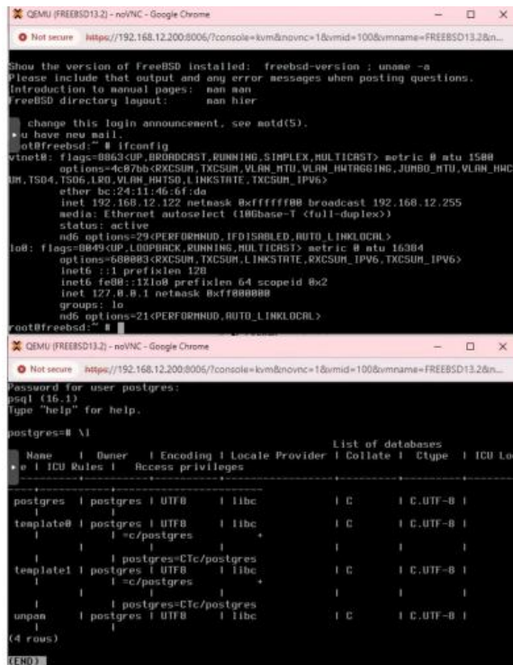
Gambar 2 Hasil Instalasi PostgreSQL 16 Pada FreeBSD 13.
