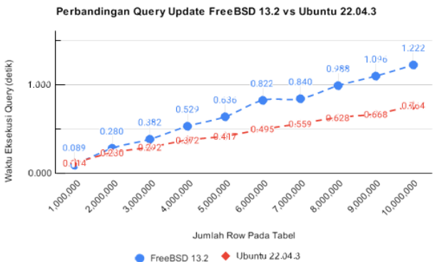
Gambar 5 Perbandingan Query Update FreeBSD 13.2 vs Ubuntu 22.04.3
