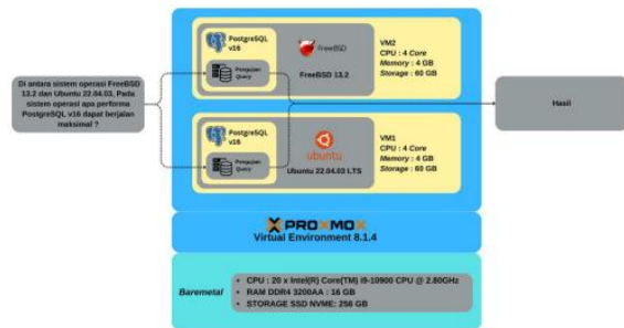
Gambar 2 Desain Implementasi Teknis Penelitian
