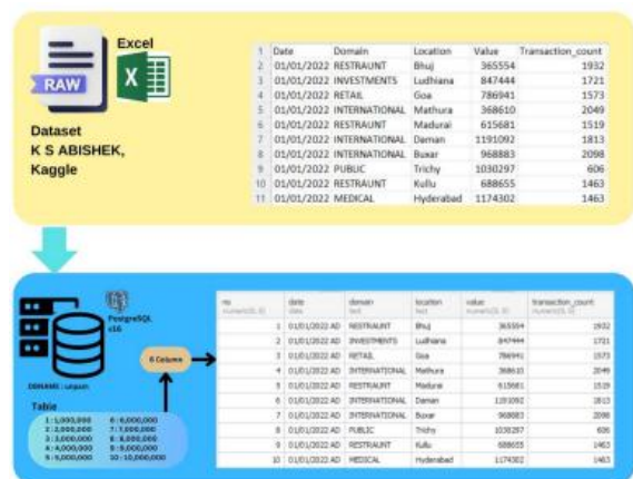
Gambar 7 Transformasi Data
